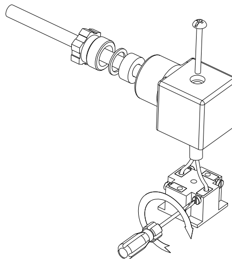
Figura 2 - Collegamento fili
